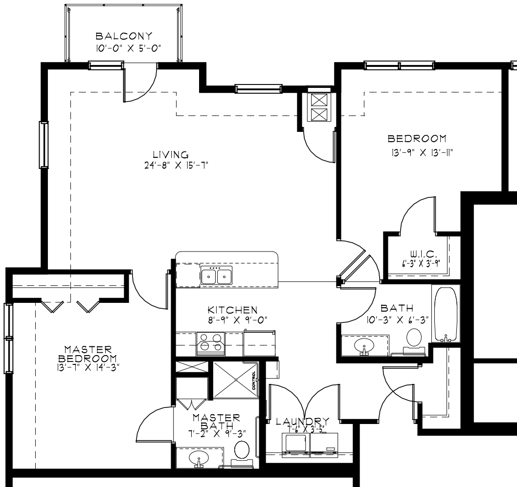
STERLING B TYPE 'B' 1266 S.F. 2 BEDROOM (1) TOTAL
